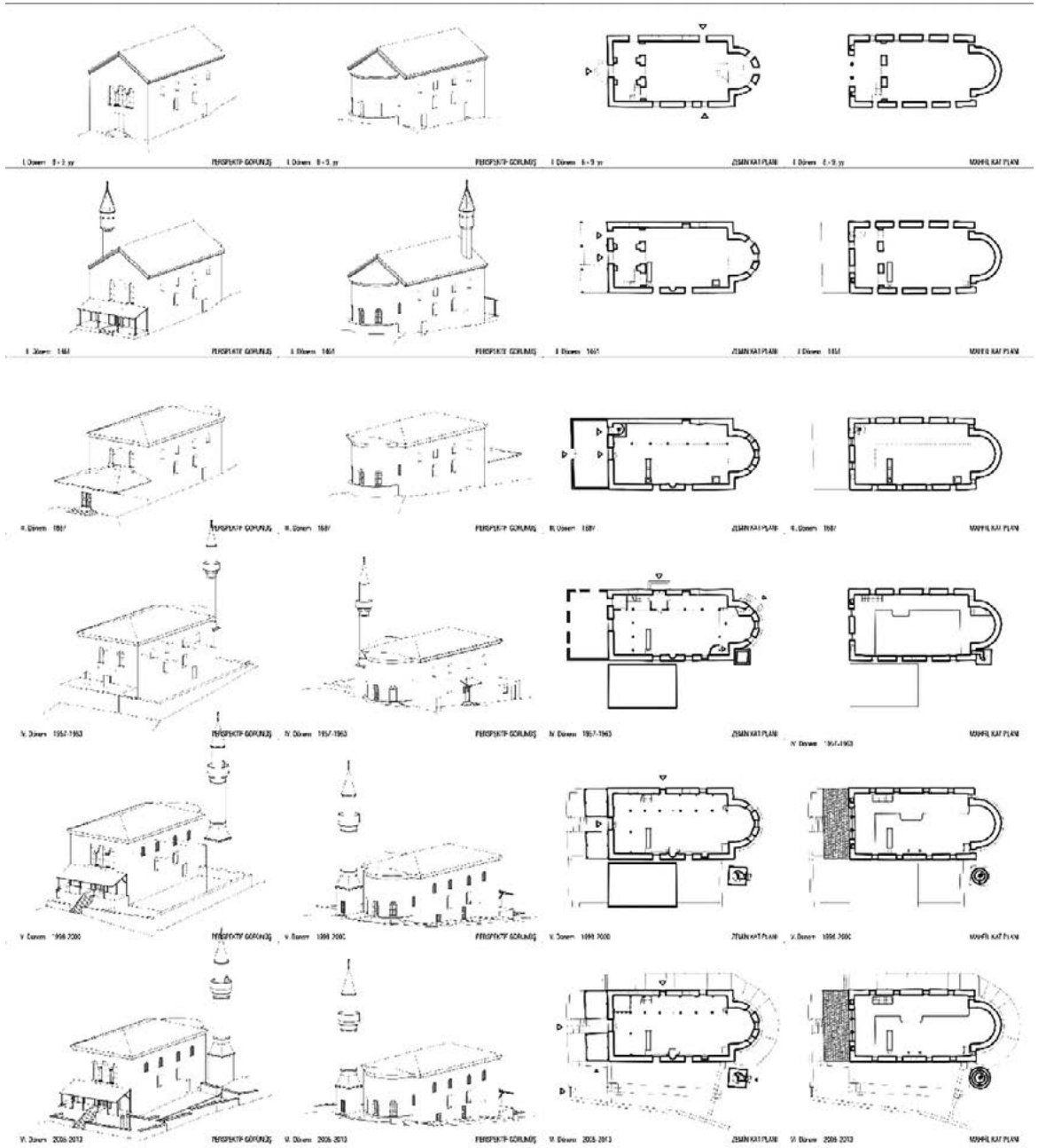
Şekil 5. Fatih Câmii restitüsyon denemesi (Asır Proje, 2021)
